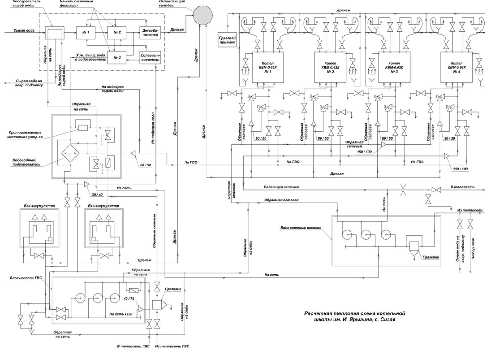
Рисунок 7 – Технологическая схема Котельной МБОУ КСОШ МУП «ШТЭС» с. Сизяя (ул. Ленина, 86а)
