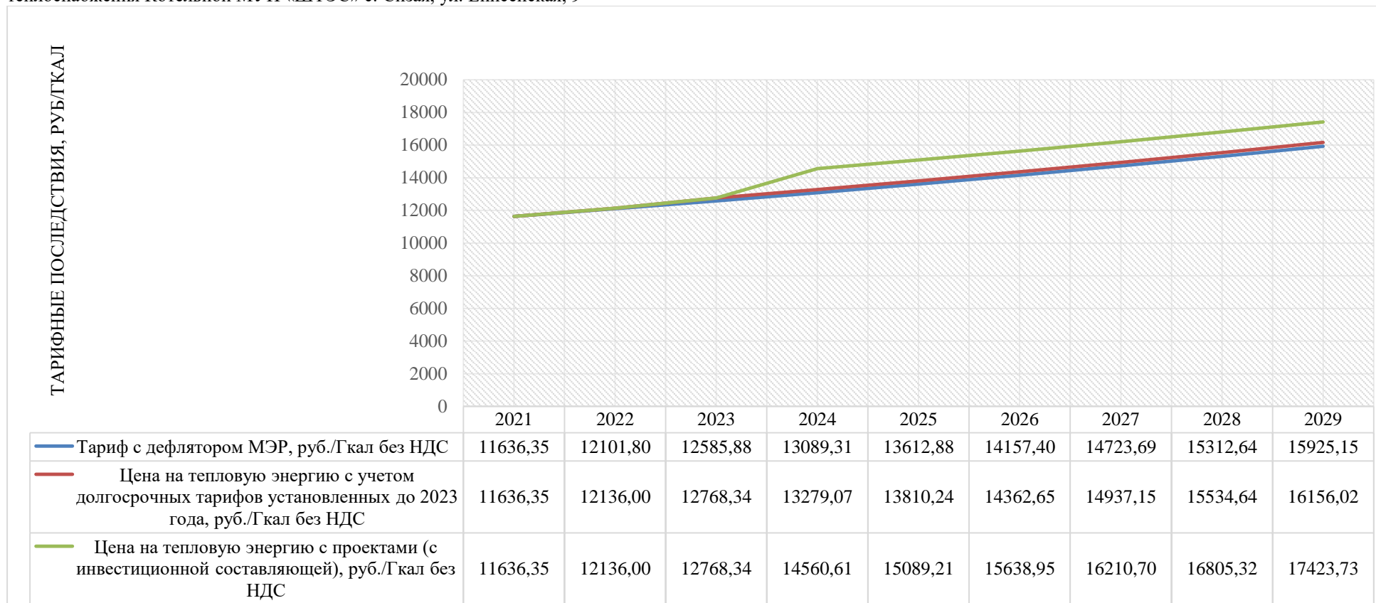
Рисунок 23 – Диаграмма ценовых последствий для потребителей Сизинского сельсовета с учетом проектов развития схемы теплоснабжения в части системы теплоснабжения Котельной МУП «ШТЭС» с. Сизая, ул. Енисейская, 9
