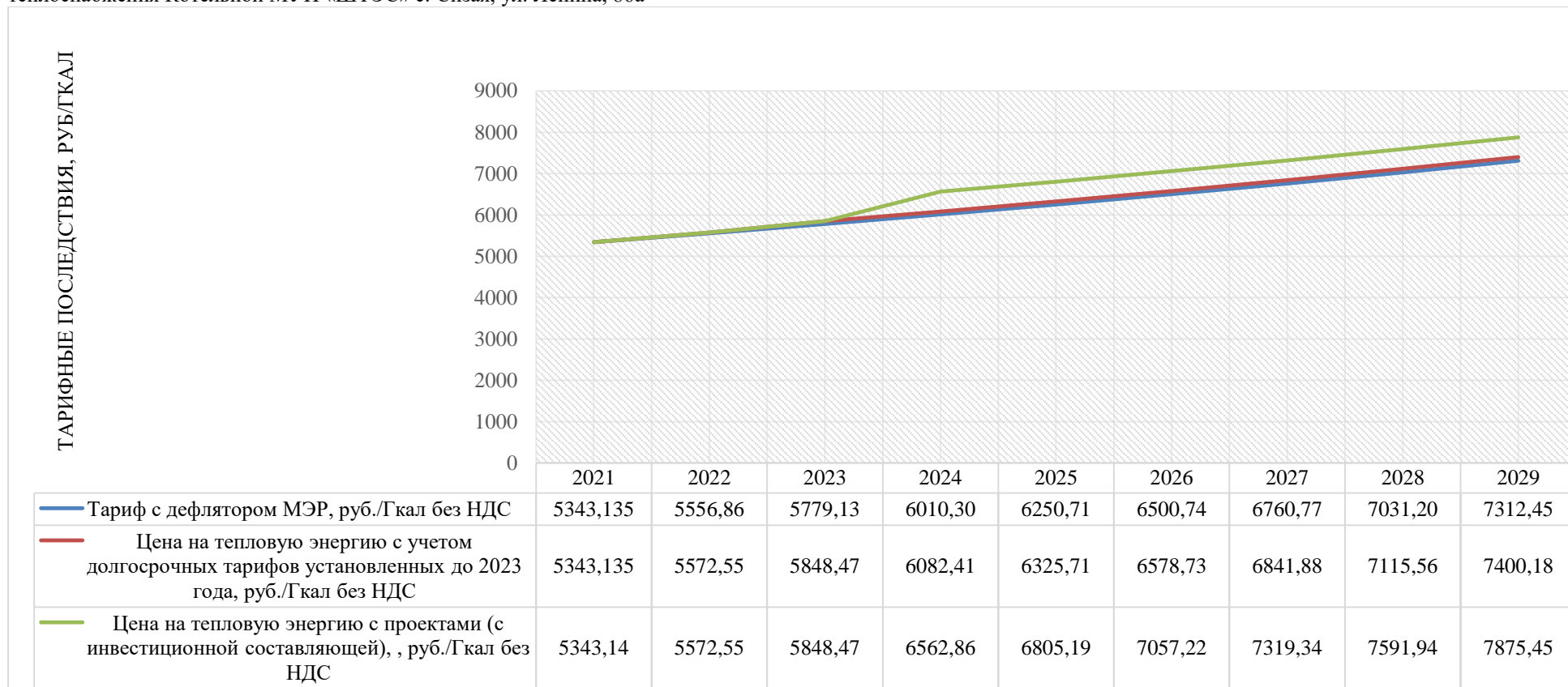
Рисунок 24 – Диаграмма ценовых последствий для потребителей Сизинского сельсовета с учетом проектов развития схемы теплоснабжения в части системы теплоснабжения Котельной МУП «ШТЭС» с. Сизая, ул. Ленина, 86а
