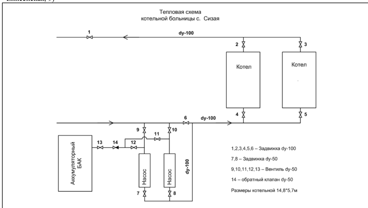
Рисунок 8 – Технологическая схема Котельной КГБУЗ «Шушенская РБ» МУП «ШТЭС» с. Сизая (ул. Енисейская, 9)
