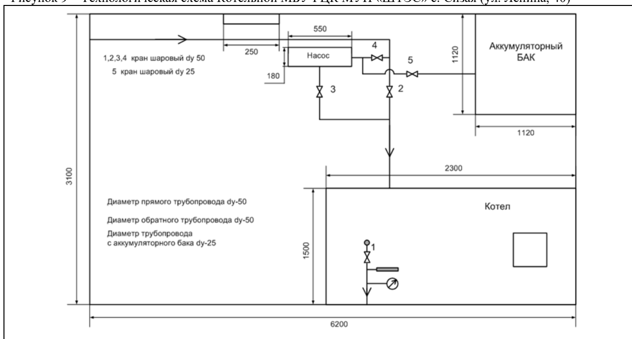
Рисунок 9 – Технологическая схема Котельной МБУ РЦК МУП «ШТЭС» с. Сизая (ул. Ленина, 40)
