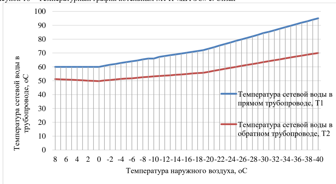
Рисунок 10 – Температурный график котельных МУП «ШТЭС» с. Сизая
