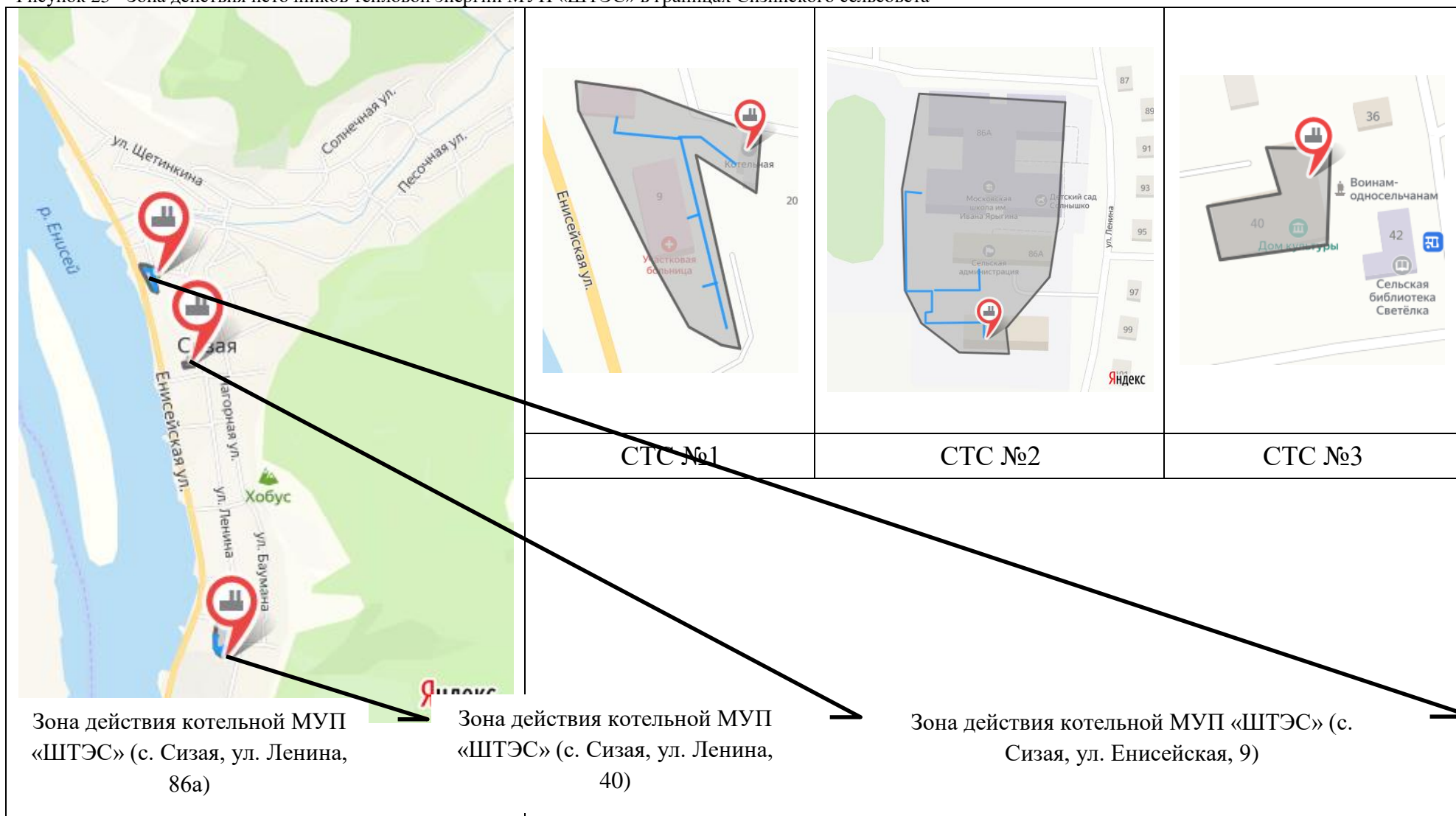
Рисунок 25 - Зона действия источников тепловой энергии МУП «ШТЭС» в границах Сизинского сельсовета
